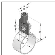
Łącznik-ucho z gwintem wewnętrznym
